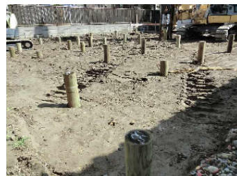
杭打ち工事
